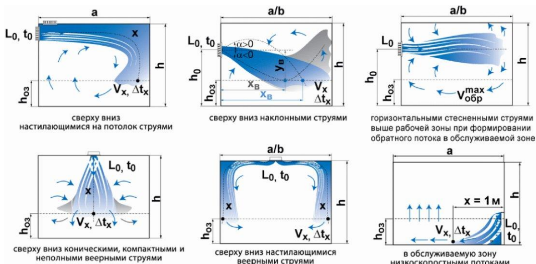
Рисунок Ж.1 - Основные схемы подачи приточного воздуха
