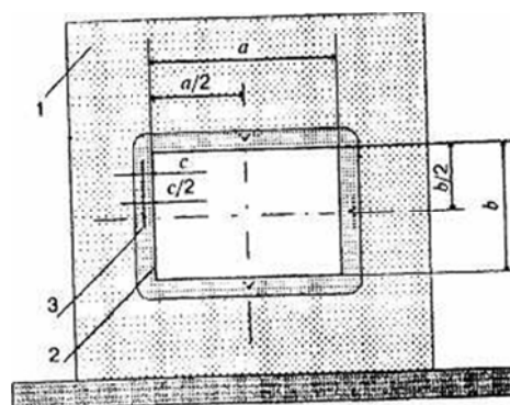
Рисунок А. 2 -Схема размещения вертикальных воздухопроводов на испытательном стенде
