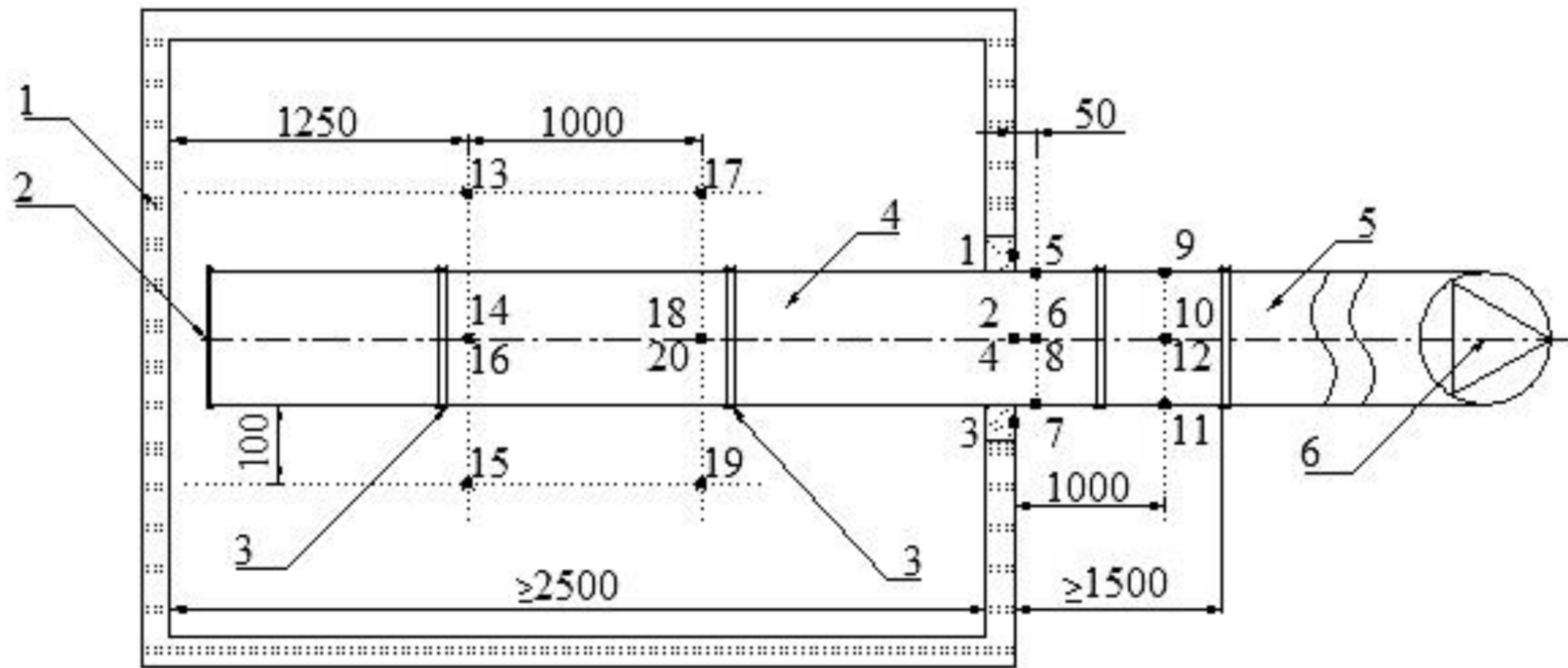
Схемы размещения воздухопроводов на испытательном стенде
