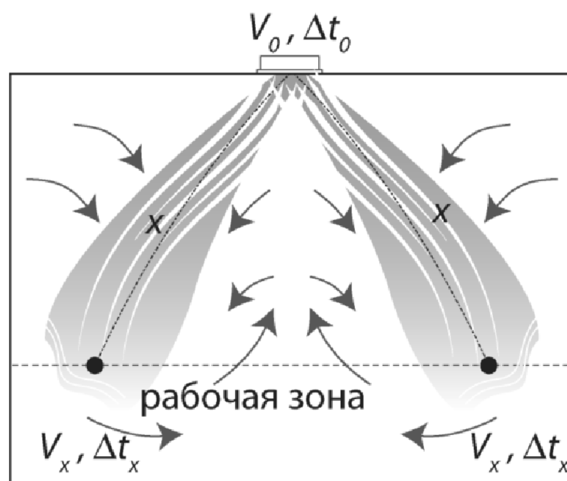
Сверху вниз коническими несмыкающимися струями
