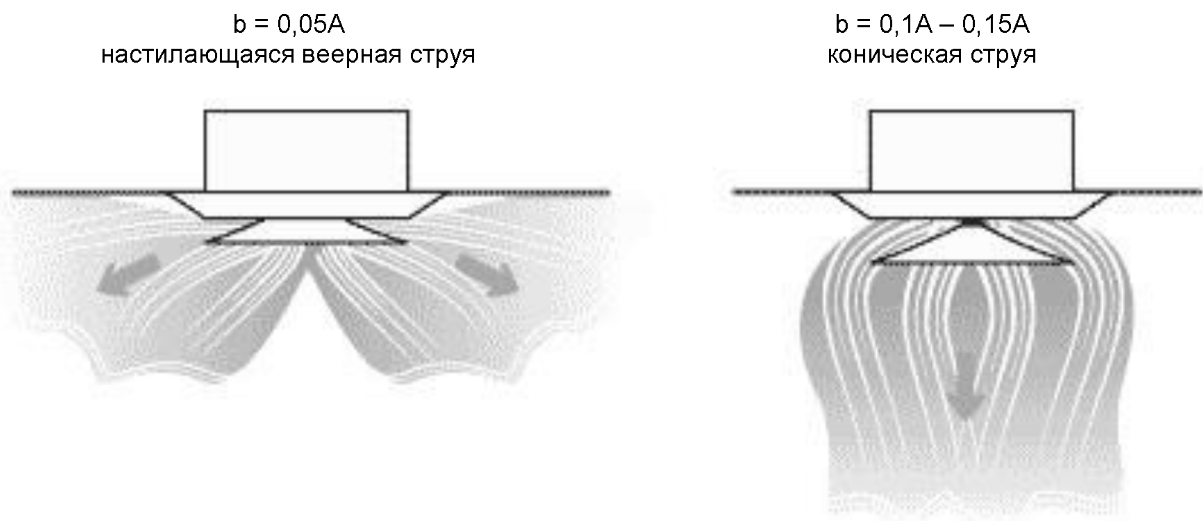
Рисунок 2 – Схемы струй, формируемых диффузором
