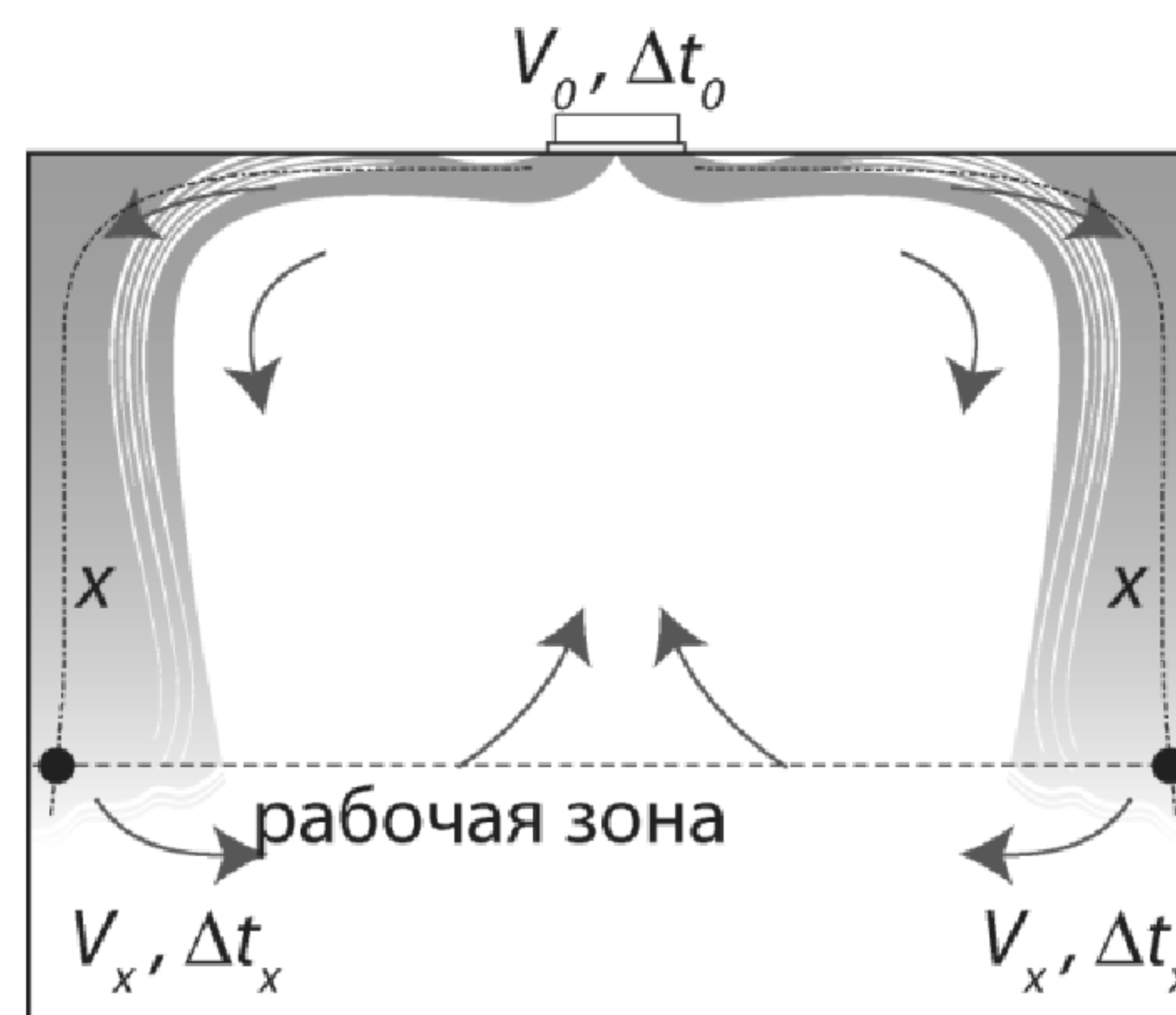
Сверху вниз настилающимися на поверхность веерными струями
