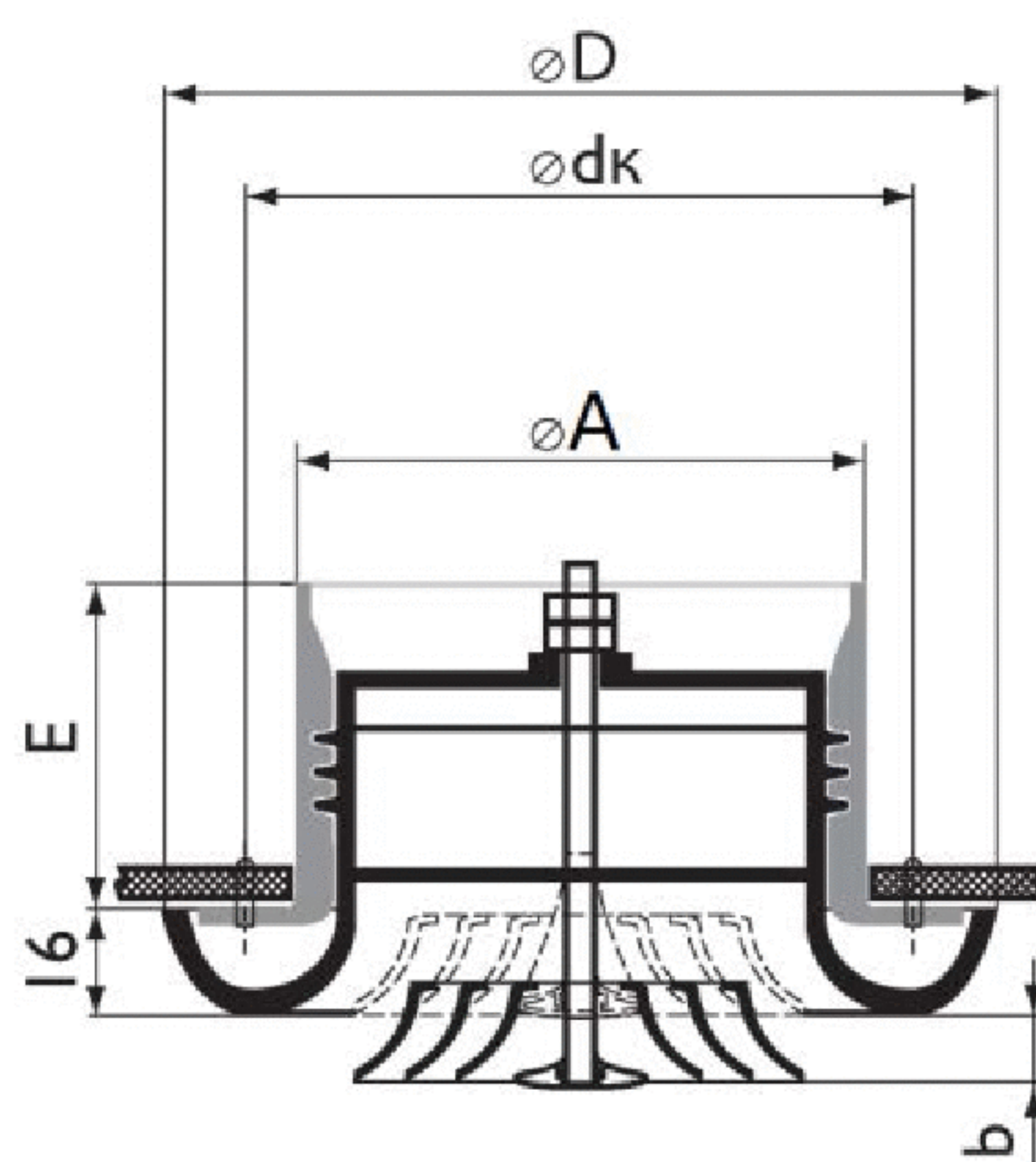
Рисунок 1 – Конструктивная схема диффузора веерного
