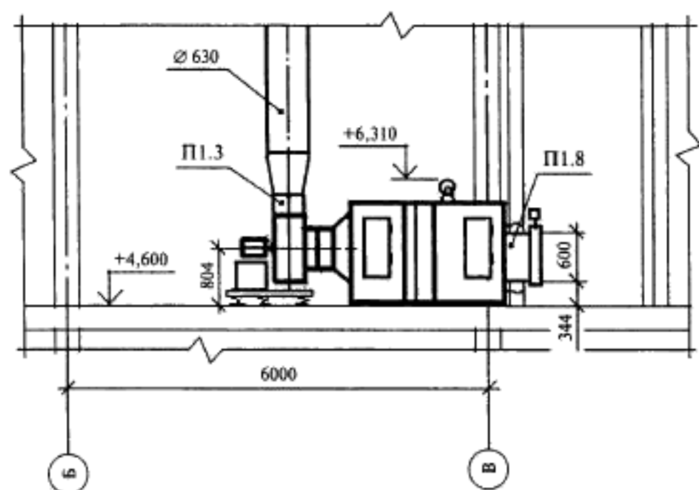
Разрез 1—1
